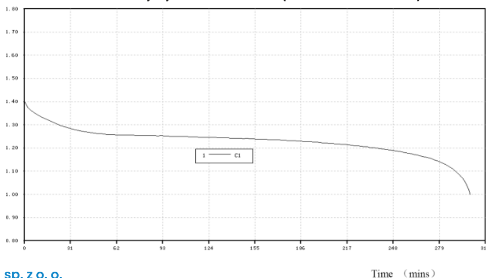
Charakterystyka rozładowania (load 0.2C - 1900 mA):
